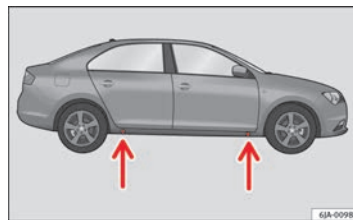
Fig. 132 Mudança de roda: pontos de apoio do macaco
