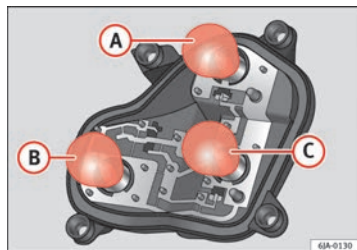
Fig. 159 Localização das lâmpadas de incandescência no porta-lâmpadas
