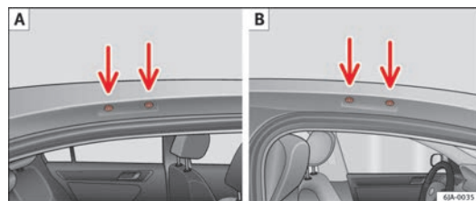
Fig. 82 Pontos de fixação das barras do tejadilho básicas
