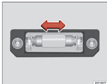
Fig. 166 Substituição de lâmpadas
