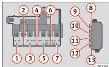
Fig. 143 Vista esquemática de fusíveis no compartimento do motor: variante 2
