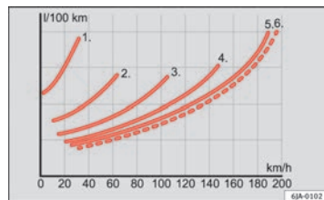
Fig. 112 Consumo de combustível em l/100 km em relação à mudança engrenada
