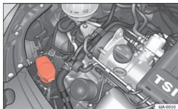
Fig. 121 Compartimento do motor: Depósito do sistema limpa-vidros
