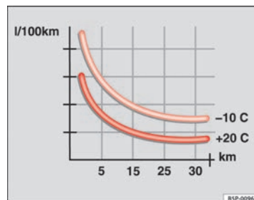
Fig. 113 Consumo de combustível em l/100km a diferentes temperaturas
