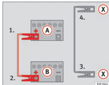
Fig. 137 Ajuda de arranque em veículos com sistema de START-STOP
