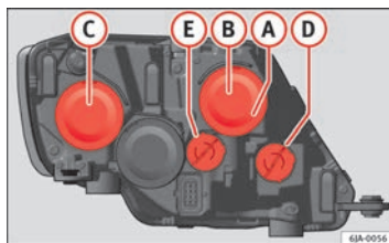
Fig. 146 Lâmpadas do farol principal
