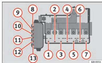
Fig. 142 Vista esquemática de fusíveis no compartimento do motor: variante 1
