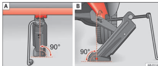
Fig. 133 colocação do macaco
