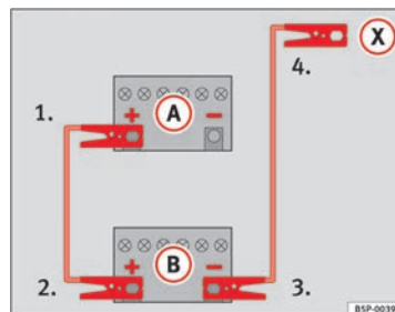
Fig. 136 Ajuda no arranque com recurso à bateria de outro veículo: A – bateria descarregada, B – bateria auxiliar
