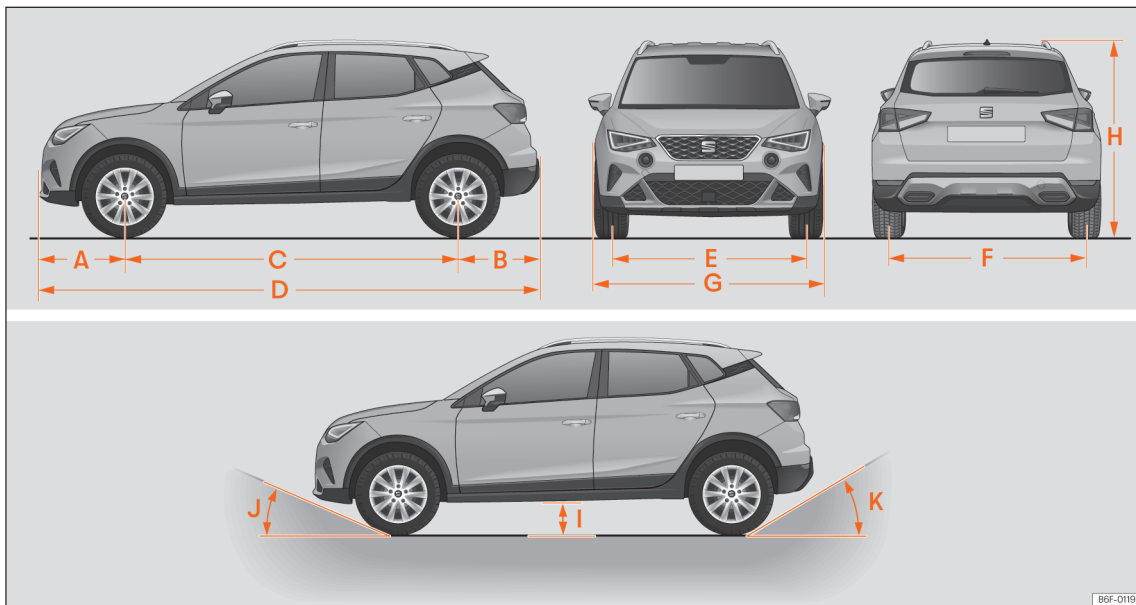
Fig. 202 Dimensões e ângulos.
