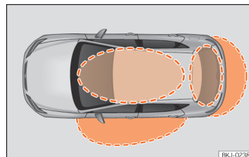
Fig. 50 Keyless Access: zonas de proximidade.
