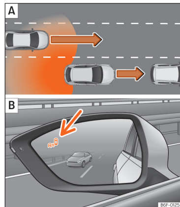
Fig. 115 Esquema: A Ultrapassagem com trânsito na parte traseira. B Indicação do assistente de mudança de faixa no lado esquerdo.
