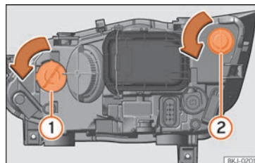
Fig. 57 No compartimento do motor: lâmpada de luz indicadora de mudança de direção ① e lâmpada de luz DRL (luz diurna) ②.
