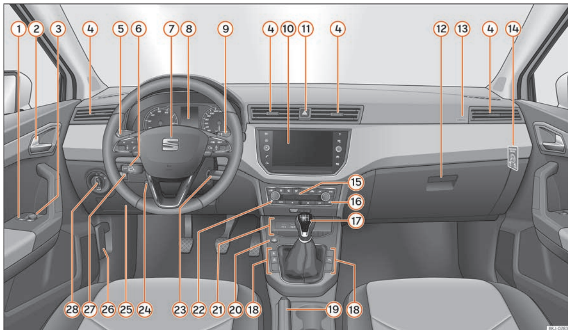
Fig. 66 Posto de condução.
