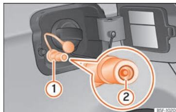
Fig. 262 Tampa do depósito aberta: bocal de enchimento de gás ①, retentor do bocal de enchimento ②.
