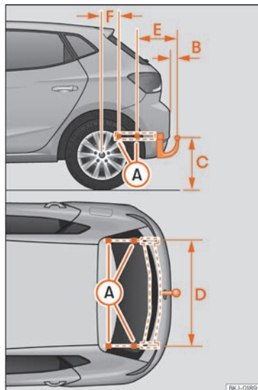
Fig. 260 Quotas e pontos de fixação para a montagem posterior de um dispositivo de reboque.
