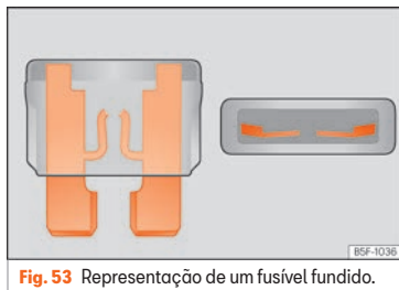
Fig. 53 Representação de um fusível fundido.
