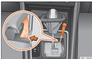
Fig. 218 Alavanca seletora: desbloqueio de emergência a partir da posição de estacionamento.
