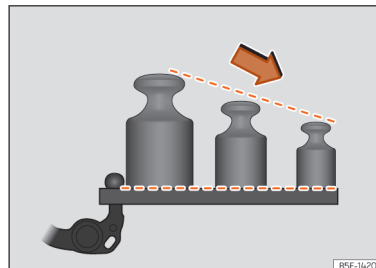
Fig. 144 Distribuição recomendada do peso no sistema de carga traseiro.
