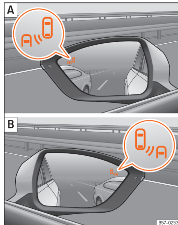
Fig. 161 Luz de controlo do assistente de mudança de faixa.
