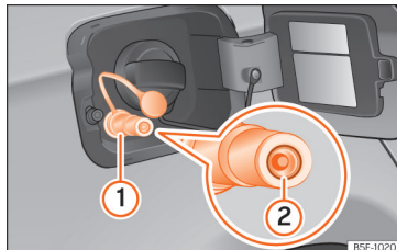
Fig. 182 Tampa do depósito aberta: bocal de enchimento de gás ①, retentor do bocal de enchimento ②.
