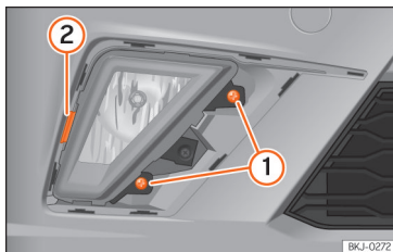
Fig. 53 Farol de nevoeiro: desmontar o porta-lâmpadas
