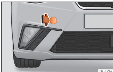
Fig. 45 Parte direita do para-choques dianteiro: retirar a tampa.
