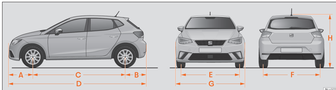
Fig. 200 Dimensões
