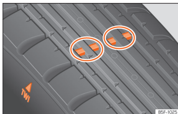
Fig. 197 Perfil do pneu: indicadores de desgaste.
