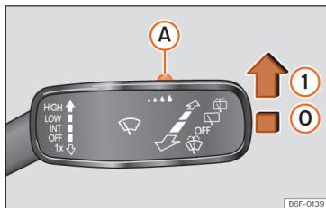
Fig. 102 Manípulo do limpador para-brisas: ajustar o sensor de chuva (A).
