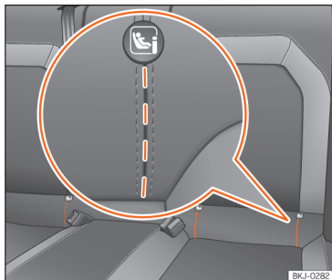
Fig. 35 Banco traseiro: ranhuras recortadas para aceder aos anéis de fixação ISOFIX/i-Size.
