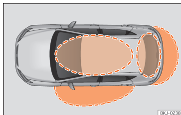
Fig. 47 Keyless Access: zonas de proximidade.
