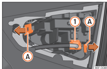
Fig. 173 desmontar o porta-lâmpadas.
