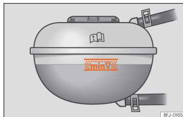
Fig. 179 No compartimento dianteiro: marca no depósito de expansão do líquido de refrigeração.
