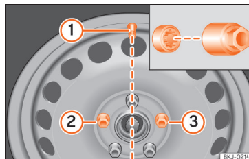
Fig. 196 Troca de roda: válvula do pneu ① e local de montagem do parafuso da roda antirroubo ② ou ③.
