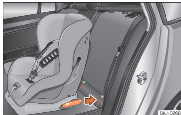
Fig. 36 Bancos traseiros: colocação da cadeira de criança com sistema ISOFIX.
