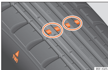
Fig. 189 Perfil do pneu: indicadores de desgaste.
