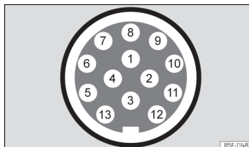
Fig. 149 Representação esquemática: atribuição dos pinos da tomada de corrente para reboque.
