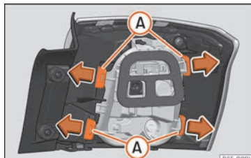
Fig. 52 Linguetas de fixação na parte posterior da unidade de luz traseira.
