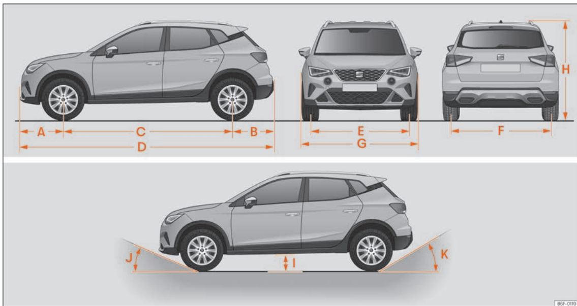
Fig. 206 Dimensões e ângulos.
