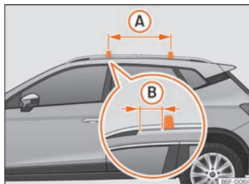
Fig. 113 Pontos de fixação das barras longitudinais para a bagageira do tejadilho.
