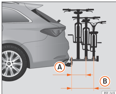
Fig. 206 Representação esquemática da saliência máxima da carga num porta-bicicletas para duas ou três bicicletas.
