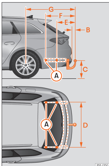
Fig. 207 Quotas e pontos de fixação para a montagem posterior de um dispositivo de reboque.
