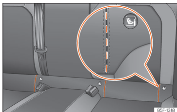
Fig. 43 Banco traseiro: ranhuras recortadas para aceder aos anéis de fixação ISOFIX/i-Size.
