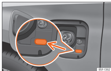
Fig. 62 Por trás da tampa da tomada de carregamento da bateria: indicador do processo de carregamento.
