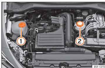
Fig. 226 Compartimento do motor: Depósitos do líquido de refrigeração
