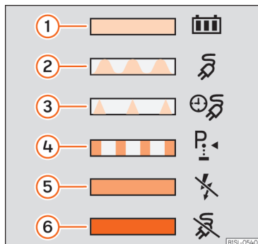
Fig. 63 Na face interior da tampa da tomada de carregamento da bateria: autocolante com informação sobre o indicador do processo de carregamento.
