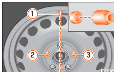
Fig. 247 Troca de roda: válvula do pneu ① e local de montagem do parafuso da roda antirroubo ② ou ③.
