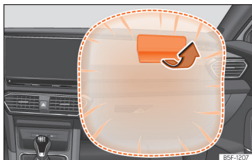
Fig. 30 Airbag do passageiro no painel de instrumentos.
