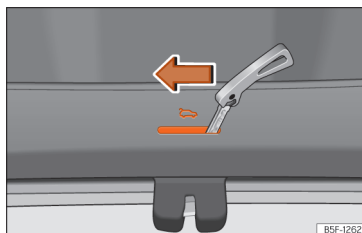
Fig. 84 Pormenor da bagageira: destrancagem de emergência (Leon).
