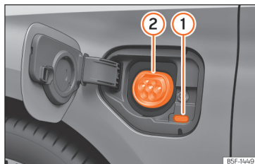
Fig. 61 Por trás da tampa de carregamento da bateria na parte dianteira esquerda: tomada de carregamento.
