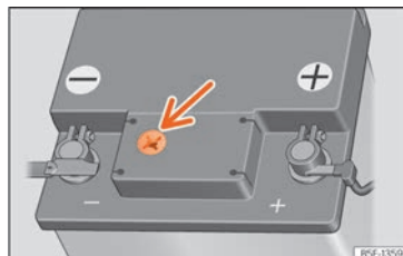
Fig. 196 Janela de inspeção na parte superior da bateria de 12 volts (representação esquemática).
