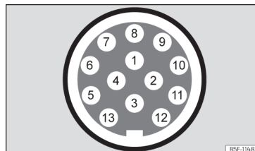
Fig. 170 Esquema: atribuição dos pinos da tomada de corrente para reboque.
