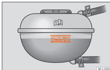
Fig. 171 No compartimento dianteiro: marca no depósito de expansão do líquido de refrigeração.
