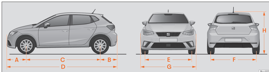
Fig. 197 Dimensões
