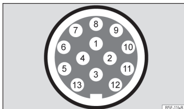
Fig. 143 Representação esquemática: atribuição dos pinos da tomada de corrente para reboque.
