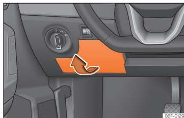
Fig. 159 No painel de instrumentos do lado do condutor: tampa da caixa de fusíveis.
