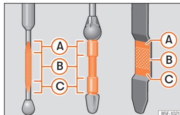
Fig. 213 Vareta de medição do nível de óleo.
