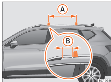
Fig. 129 Pontos de fixação das barras longitudinais para a bagageira do tejadilho.
