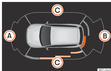
Fig. 191 Visualização do auxiliar de estacionamento no ecrã do sistema de infotainment.
