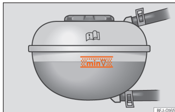
Fig. 215 No compartimento do motor: marca no depósito de expansão do líquido de refrigeração.
