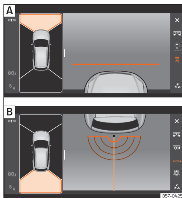
Fig. 200 Visualização no ecrã do sistema de visão periférica: A) Câmara dianteira: vista todo-o-terreno. B) Câmara traseira: vista todo-o-terreno.
