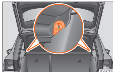
Fig. 117 Na bagageira: desmontar e montar a chapeleira.
