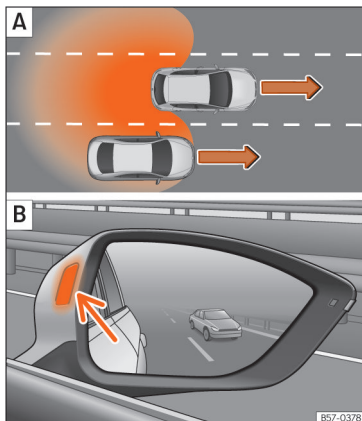
Fig. 181 Esquema: A ) Situação numa ultrapassagem e incorporação posterior na via de circulação direita. B ) Indicação do assistente de mudança de faixa no retrovisor exterior direito.
