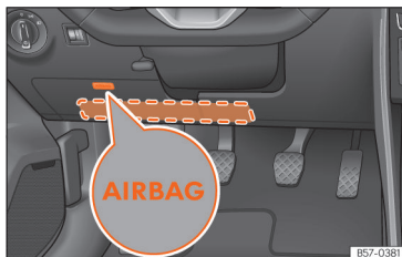
Fig. 18 No lado do condutor: localização do airbag de joelhos.
