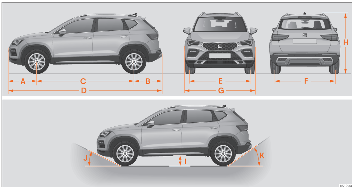
Fig. 225 Dimensões
