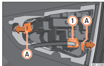
Fig. 174 desmontar o porta-lâmpadas.
