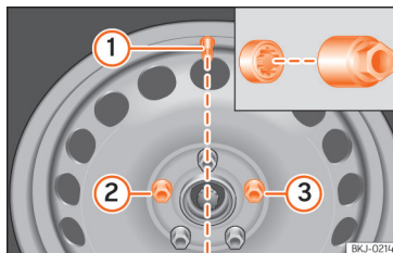
Fig. 197 Troca de roda: válvula do pneu ① e local de montagem do parafuso da roda antirroubo ② ou ③.
