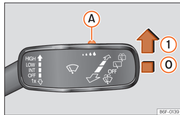
Fig. 77 Manípulo do limpa-vidros: ajustar o sensor de chuva (A).
