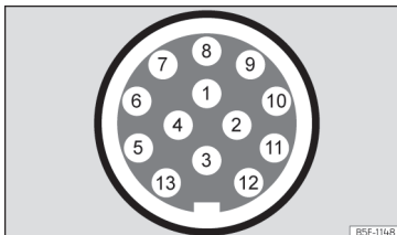
Fig. 145 Representação esquemática: atribuição dos pinos da tomada de corrente para reboque.
