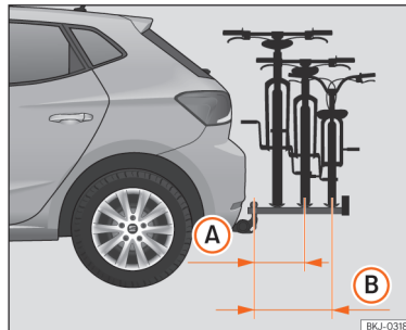
Fig. 147 Representação esquemática da saliência máxima da carga num porta-bicicletas para duas ou três bicicletas.
