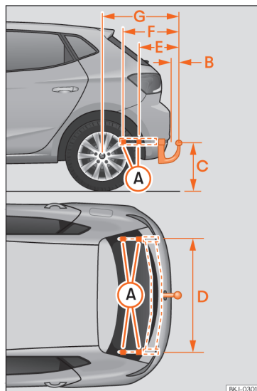
Fig. 148 Quotas e pontos de fixação para a montagem posterior de um dispositivo de reboque.
