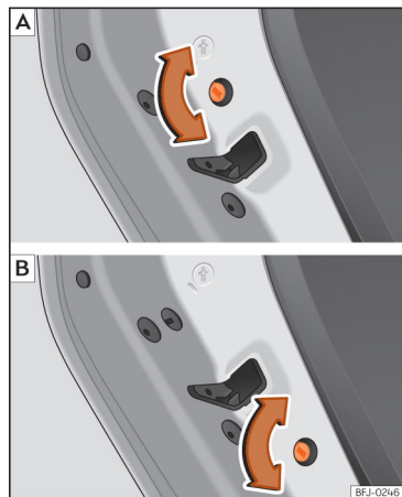
Fig. 56 Sistema de segurança para crianças da porta esquerda (simétrico na porta direita). Em função da versão ou do país, o veículo está equipado com a variante A ou a variante B .
