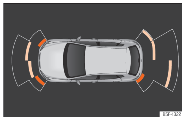
Fig. 124 Visualização do auxiliar de estacionamento no ecrã do sistema infotainment.
