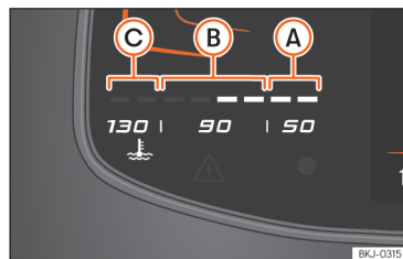
Fig. 7 Painel de instrumentos Basic: indicador da temperatura do líquido de refrigeração do motor.
